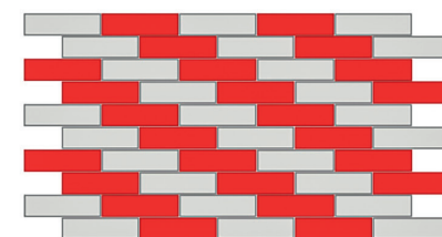
Běhounová vazba s přesunem o 1/4 cihly
