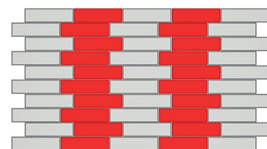
Běhounová vazba s přesunem o 1/3 cihly
