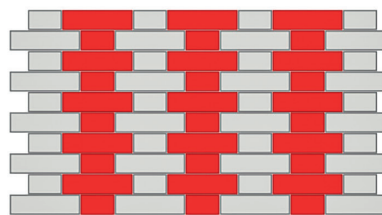
Křížová vazba typ 2
